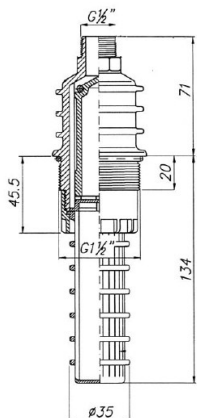
Légtelenítő és vákuumtörő szelep
